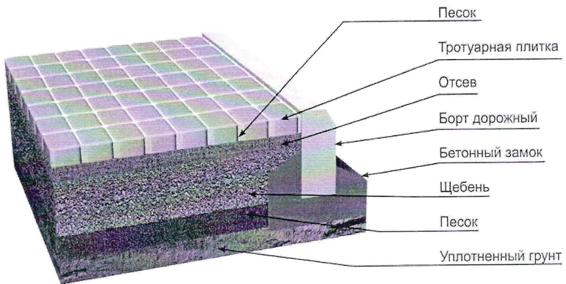
Схема 1. Схема укладки брусчатки
